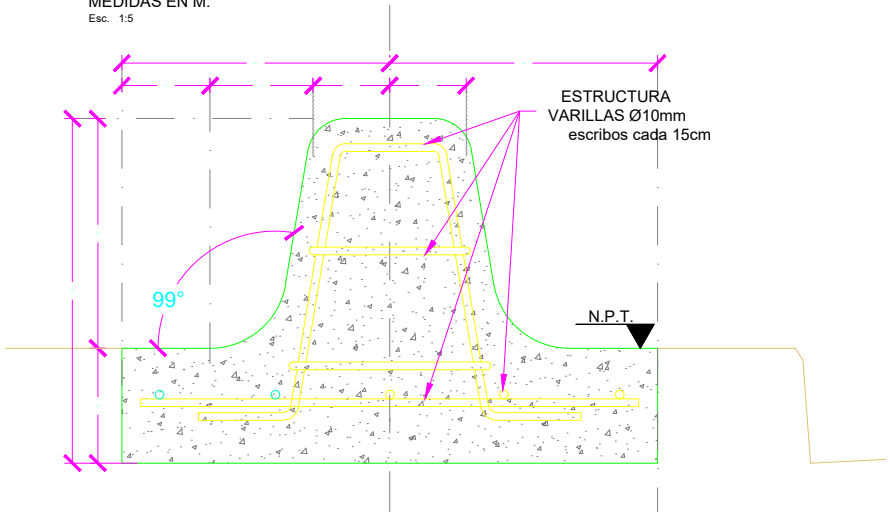
SECCION A-A BOLARDO TIPO 2 MEDIDAS EN M. Esc. 1:5
