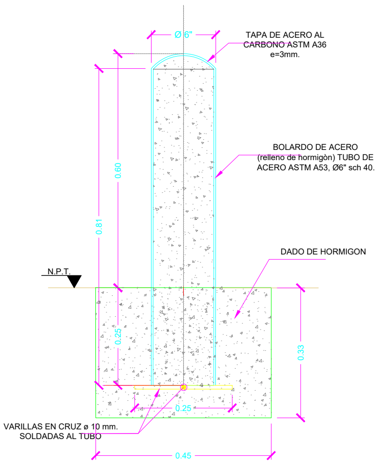
SECCION A-A BOLARDO TIPO 3A MEDIDAS EN M. Esc. 1:5
