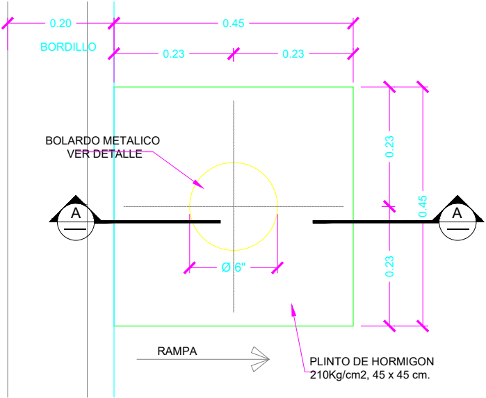
SECCION A-A BOLARDO TIPO 3A MEDIDAS EN M. Esc. 1:5
