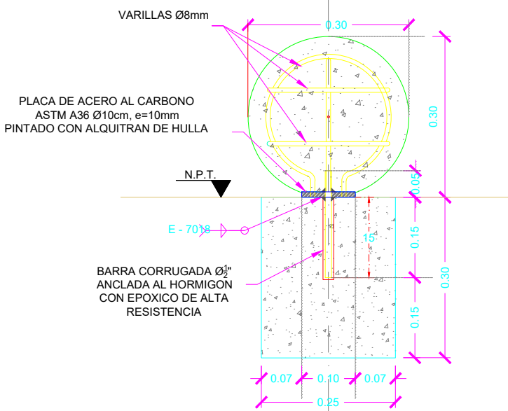
SECCION A-A BOLARDO TIPO 1 MEDIDAS EN M. Esc. 1:5
