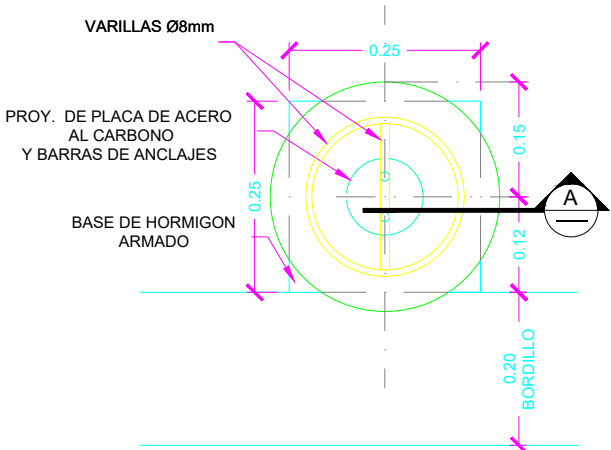
PLANTA BOLARDO TIPO 1 MEDIDAS EN M. Esc. 1:5
