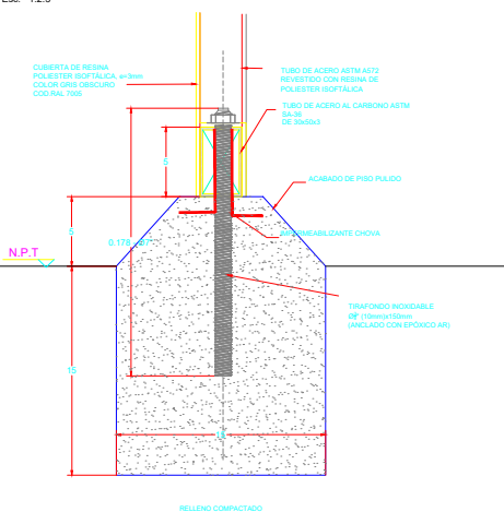
DETALLE CIMENTACION BASURERO FIBRA DE VIDRIO MEDIDAS EN M.
