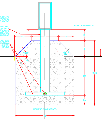
DETALLE CIMENTACION BASURERO A/I MEDIDAS EN M.
