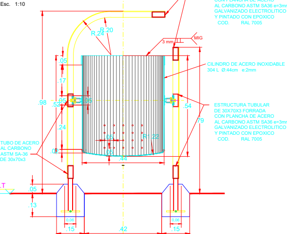
ALZADO A BASURERO ACERO INOX MEDIDAS EN M.
