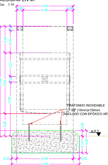
SECCION B-B BASURERO FIBRA DE VIDRIO MEDIDAS EN M.
