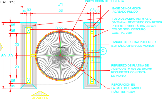
PLANTA BASURERO FIBRA DE VIDRIO MEDIDAS EN M.
