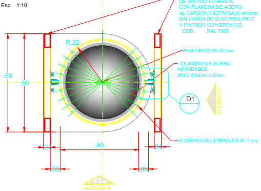
PLANTA BASURERO ACERO INOX MEDIDAS EN M.
