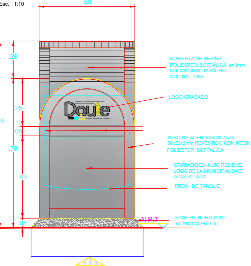
ALZADO B BASURERO FIBRA DE VIDRIO MEDIDAS EN M.
