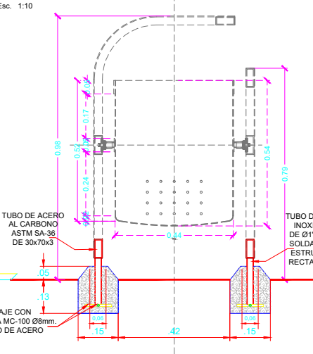
ALZADO A BASURERO ACERO INOX MEDIDAS EN M.
