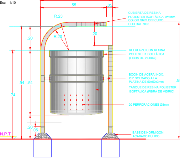
ALZADO A BASURERO FIBRA DE VIDRIO MEDIDAS EN M.
