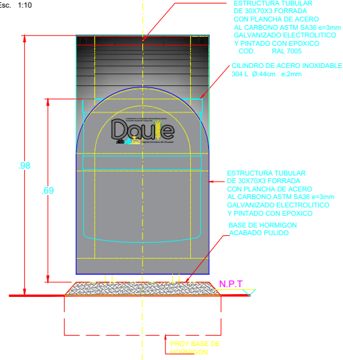
ALZADO B BASURERO ACERO INOX MEDIDAS EN M.
