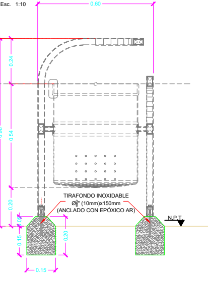
SECCION A-A BASURERO FIBRA DE VIDRIO MEDIDAS EN M.
