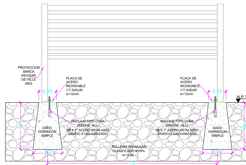
CORTE A-A BANCA TIPO MEDIDAS EN M.
