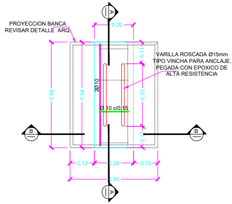
PLANTA BANCA TIPO A MEDIDAS EN M.
