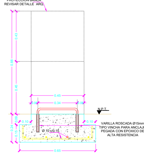
CORTE B-B BANCA TIPO 2 MEDIDAS EN M.
