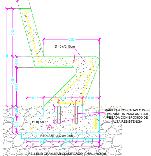
CORTE A-A BANCA TIPO 2 MEDIDAS EN M.
