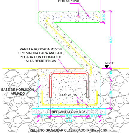
CORTE A-A BANCA TIPO A MEDIDAS EN M.
