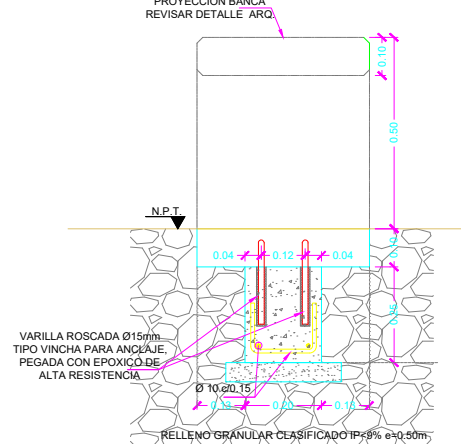
CORTE B-B BANCA TIPO A MEDIDAS EN M.
