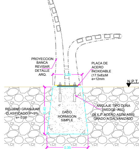
CORTE B-B BANCA TIPO 3 MEDIDAS EN M.
