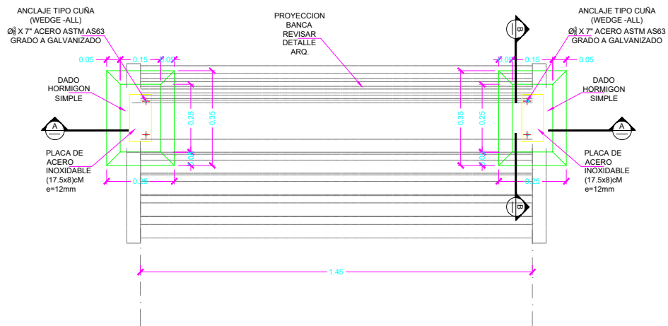
PLANTA BANCA TIPO : MEDIDAS EN M.
