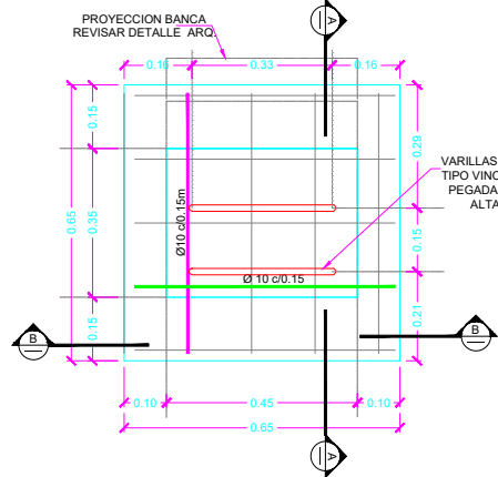
PLANTA BANCA TIPO 2 MEDIDAS EN M.
