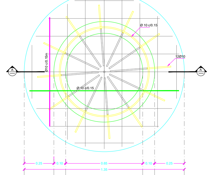
PLANTA BANCA CIRCULAR TIPO 1A MEDIDAS EN M. Esc. 1:10
