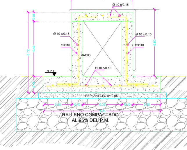
SECCION 1-1 BANCA CIRCULAR TIPO 1B MEDIDAS EN M. Esc. 1:10
