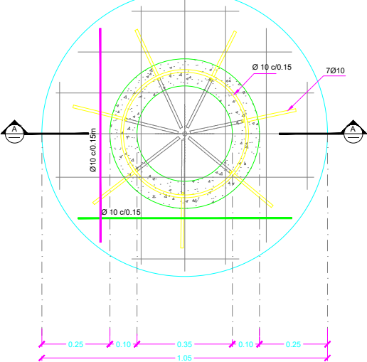
PLANTA BANCA CIRCULAR TIPO 1B MEDIDAS EN M. Esc. 1:10
