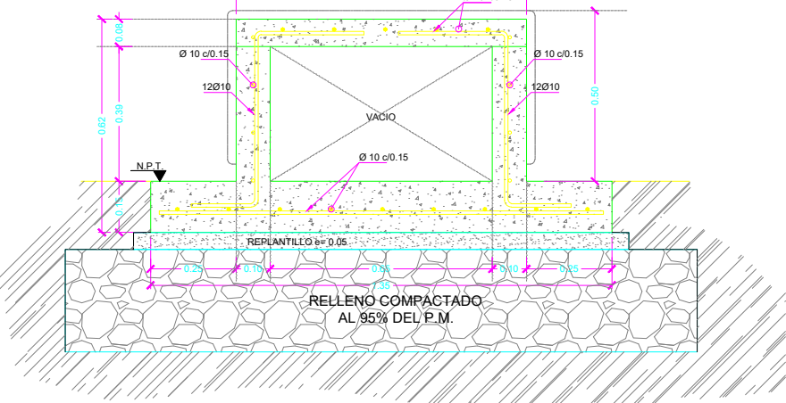
SECCION 1-1 BANCA CIRCULAR TIPO 1A MEDIDAS EN M. Esc. 1:10
