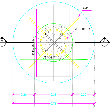
PLANTA BANCA CIRCULAR TIPO 1C MEDIDAS EN M. Esc. 1:10
