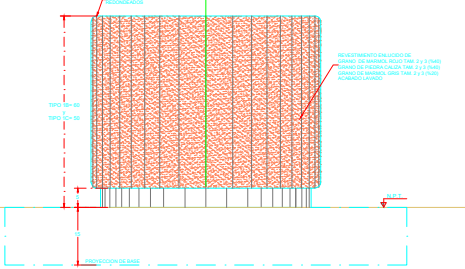
FACHADA ASIENTO TIPO 1B - 1C MEDIDAS EN M. Esc. 1:10
