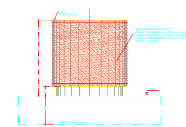
FACHADA ASIENTO TIPO 1A MEDIDAS EN M. Esc. 1:10
