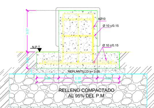
SECCION 1-1 BANCA CIRCULAR TIPO 1C MEDIDAS EN M. Esc. 1:10
