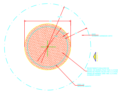
PLANTA BANCA CIRCULAR TIPO 1A MEDIDAS EN M. Esc. 1:10
