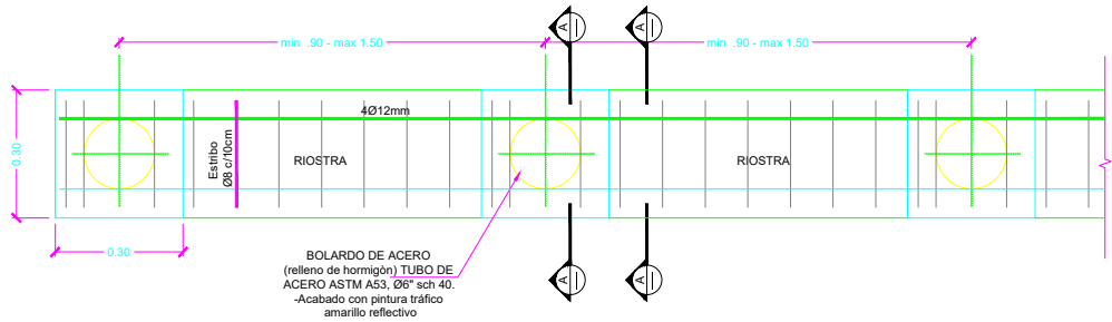
PLANTA BOLARDO TIPO 3B MEDIDAS EN M. Esc. 1:10
