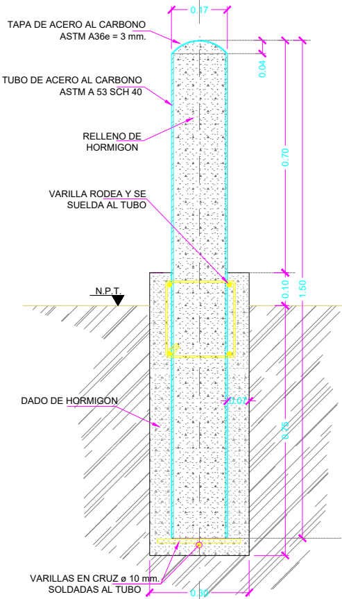
SECCION A-A TIPO 3B MEDIDAS EN M. Esc. 1:10
