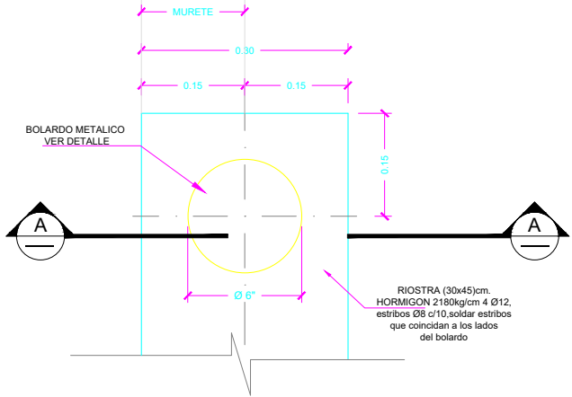
PLANTA BOLARDO TIPO 3C MEDIDAS EN M. Esc. 1:5
