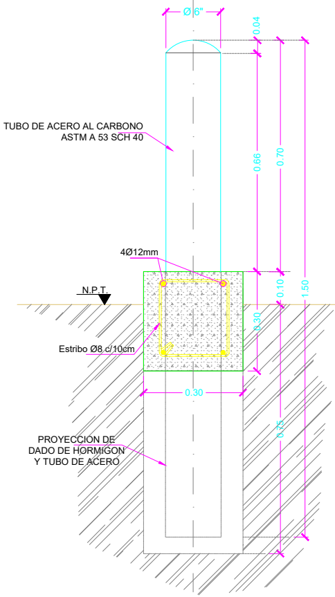
SECCION B-B TIPO 3B MEDIDAS EN M. Esc. 1:10
