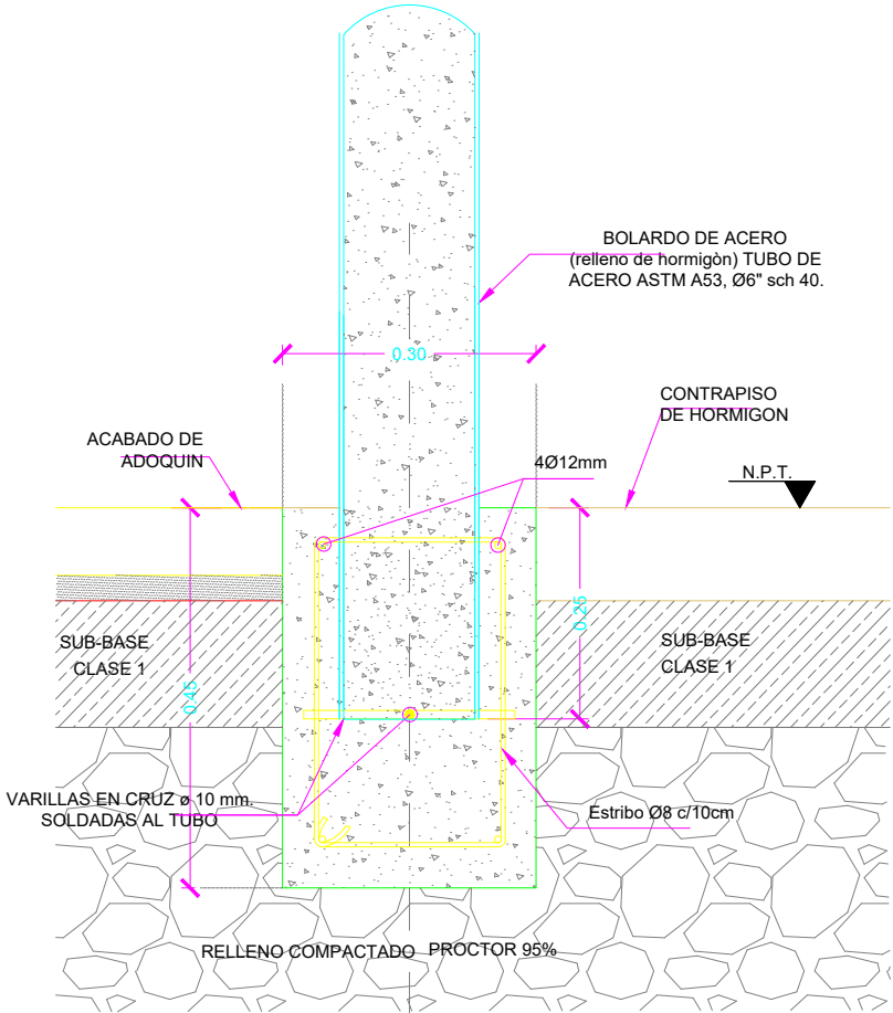
SECCION A-A BOLARDO TIPO 3C MEDIDAS EN M. Esc. 1:5
