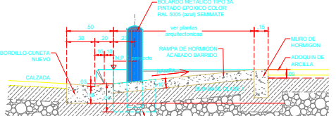
SECCION 2 Escala. 1:20
