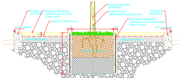
SECCION 1 Escala. 1:20
