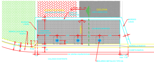
PLANTA TIPO Escala. 1:50
