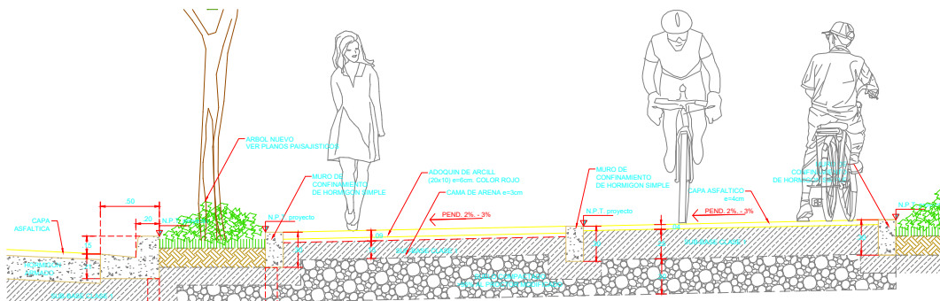
SECCION TIPO Escala. 1:20
