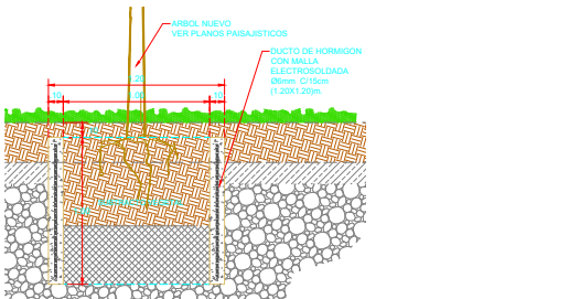
SECCION TIPO en Area de Paisajismo y Contemplación Escala. 1:20
