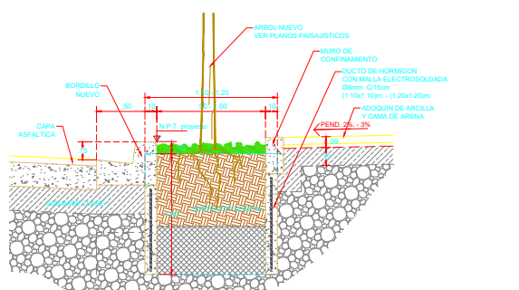
SECCION TIPO en Area de Amortiguamiento Escala. 1:20
