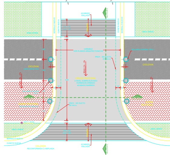
PLANTA Escala. 1:50
