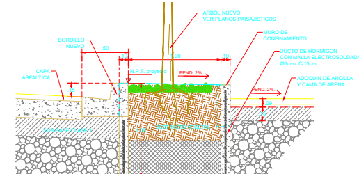
SECCION 2 Escala. 1:20
