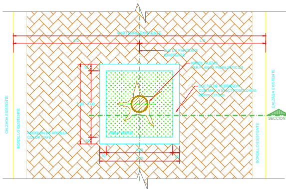
PLANTA TIPO (en parterre) Escala. 1:20
