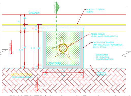
PLANTA TIPO (en Area de Estacionamiento) Escala. 1:20
