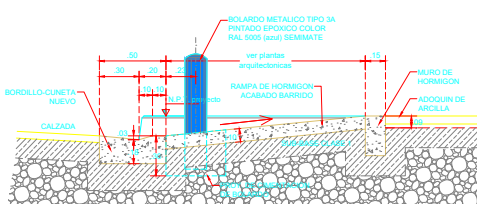
SECCION 1 Escala. 1:20
