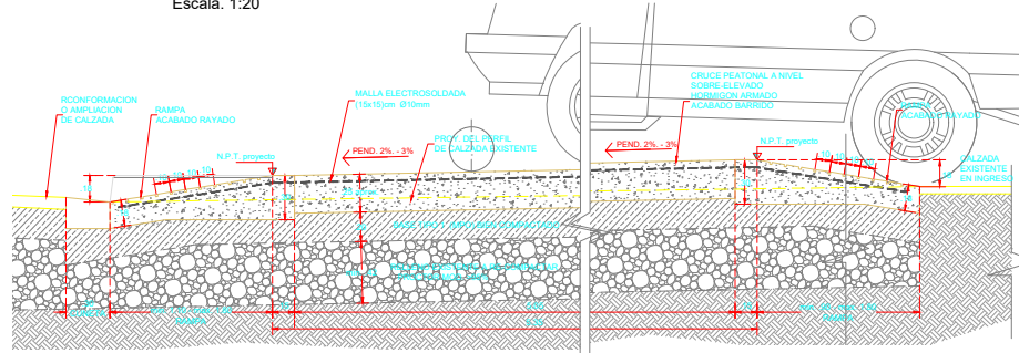
SECCION 2 Escala. 1:20
