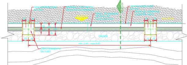
PLANTA TIPO Escala. 1:20
