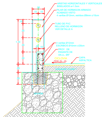
SECCION TIPO Escala. 1:20
