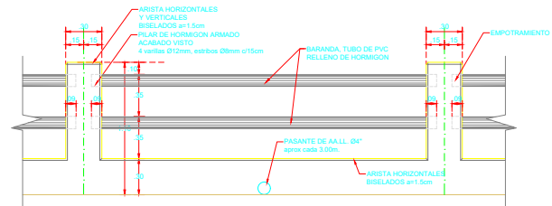
ALZADO A Escala. 1:20
