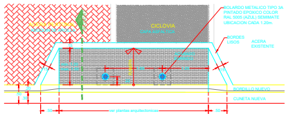
PLANTA TIPO 2 Escala. 1:50
