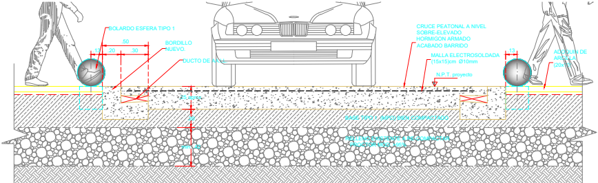
SECCION 1 Escala. 1:20
