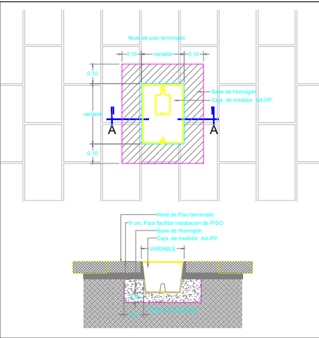
DETALLE D17B BASE DE Ho PARA ANCLAJE ESC:10
