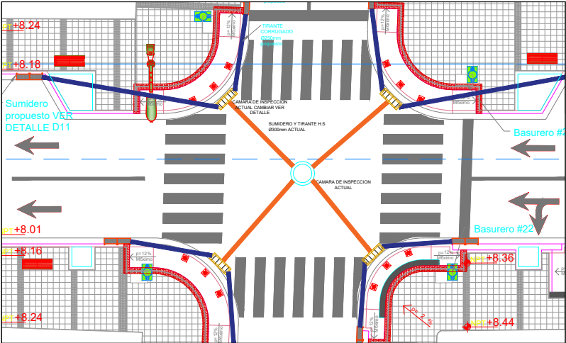
DETALLE D16 DE REJILLA DE AALL A CAMARA DE INSPECCION ESC:100
