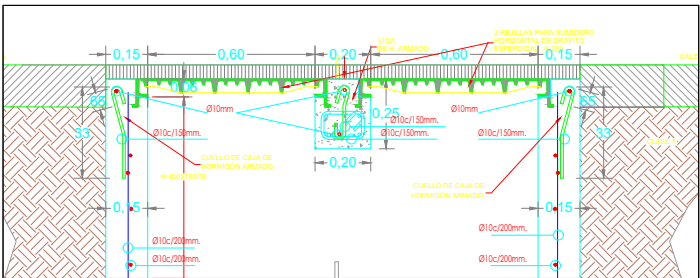
CORTE DD'
