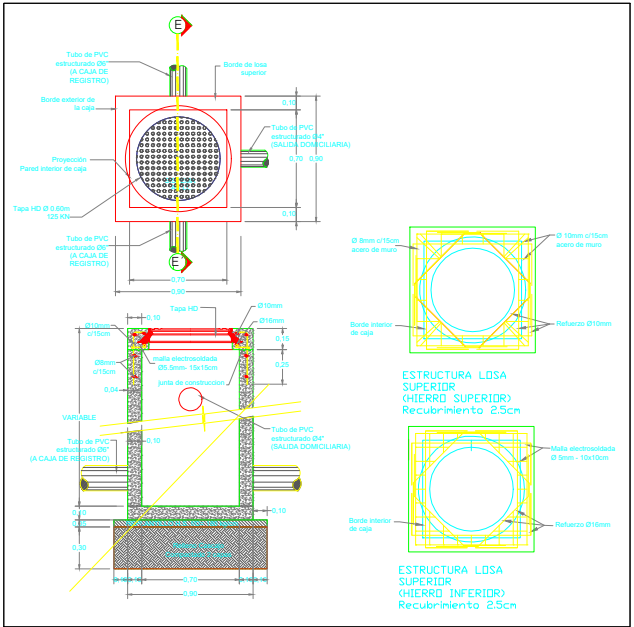
DETALLE D6 DE CAJA DE PASO AA.SS. EN ACERA ESC: 1 -20
