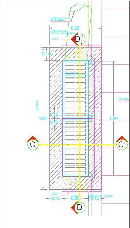
PLANTA
