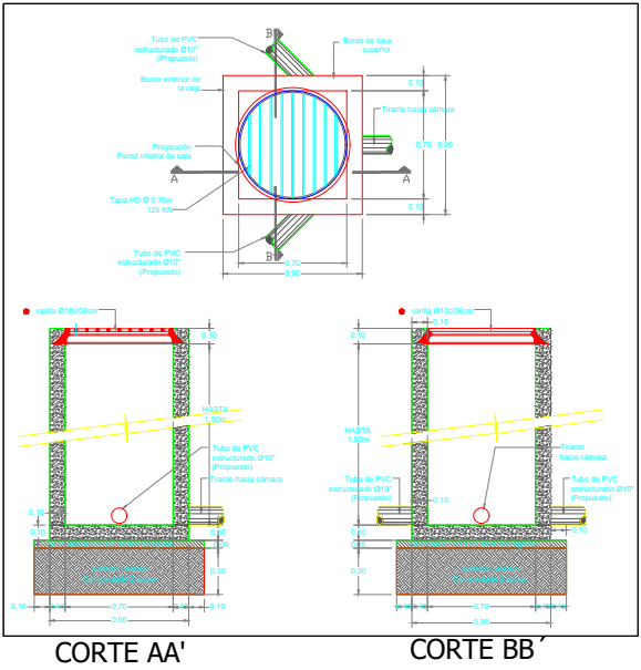
DETALLE D10 CAJA DE REGISTRO DE HoAo DE AALL A CONSTRUIRSE EN CALZADA ESC: 1 -20
