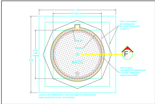
DETALLE D7 INSTALACION DE AA.SS.
